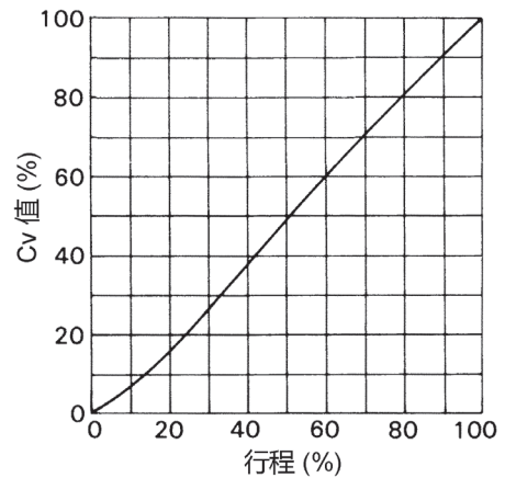
b. 线性特性 (LV 金属阀座)
