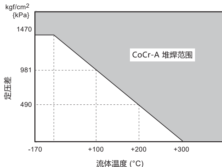
图 2. 需要 CoCr-A 堆焊的温度、压力范围
